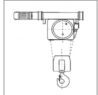
Tipo 53C1 carrello birotaia con paranco sospeso
