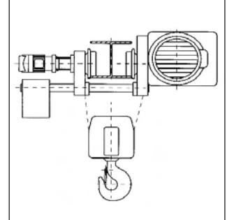
Tipo 83 carrello monotrave a ingombro ridotto
