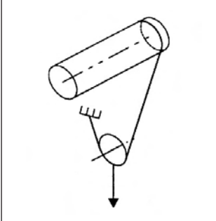
Versioni Standard S4 - a 4 tiri di fune
