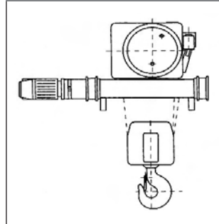
Tipo 53 carrello birotaia con paranco appoggiato
