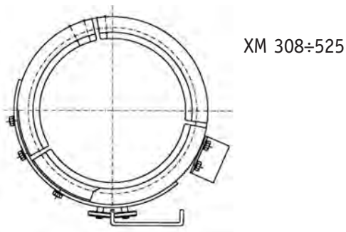
Schema guidafune con guida a rotolamento per paranchi
