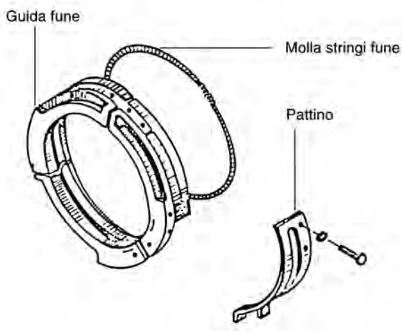
Schema guidafune con guida a rotolamento per paranchi
