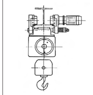
Tipo 3 carrello monotrave a ingombro normale
