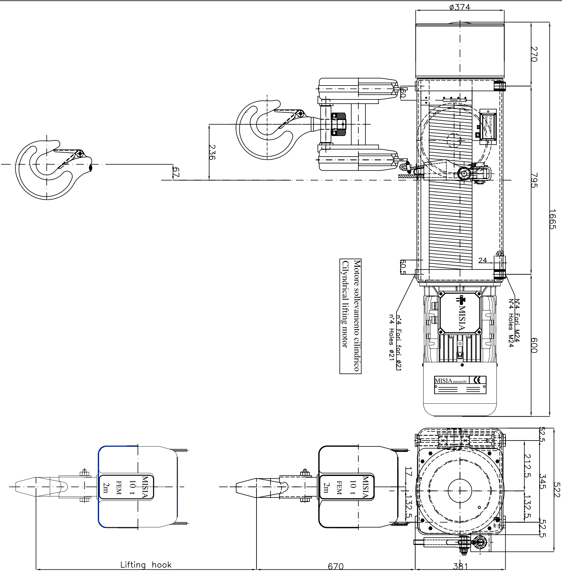
Paranco figura 5. tipo ----- Hoist type ----- XM525NS4H10A/5
