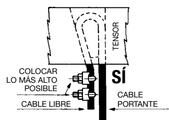
Fijación de mordazas correcta
