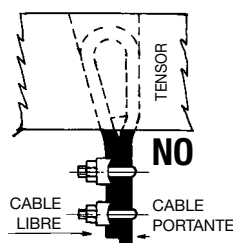
Fijación de mordazas incorrecta
