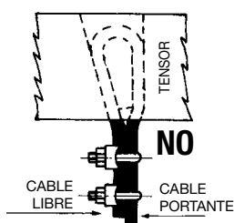
Fijación de mordazas incorrecta
