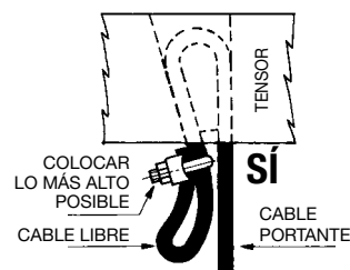
Fijación de mordazas correcta
