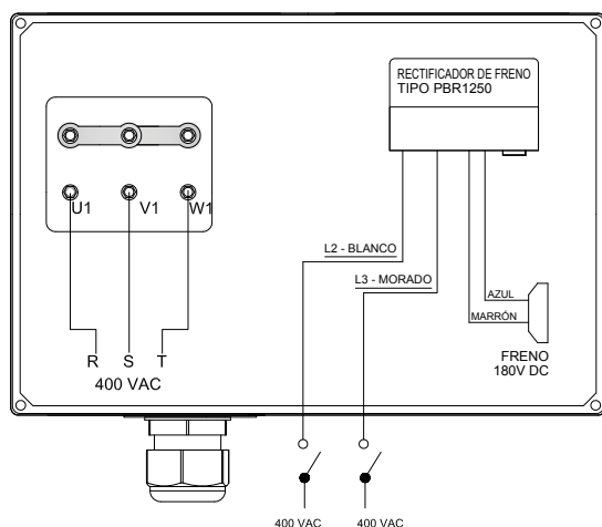
MOTOR DE VELOCIDAD ÚNICA PARA INVERSOR ALIMENTACIÓN 400V 3PH
