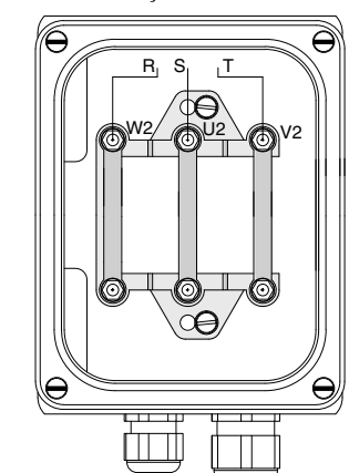
MOTOR COM DUPLA VELOCIDADE ALIMENTAÇÃO 220V 3PH
