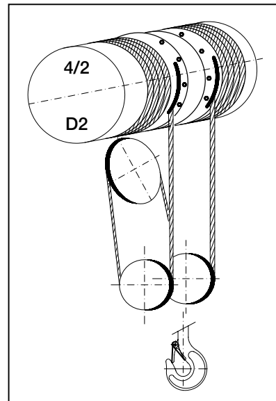
D2 - 4 TIROS DE CABLE (4/2) TIRO CENTRAL
