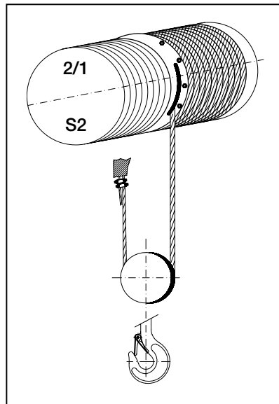
S2 - 2 TIROS DE CABLE (2/1)
