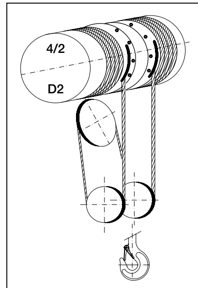
D2 - 4 TRAÇÕES DE CABO (4/2) TRAÇÃO CENTRAL
