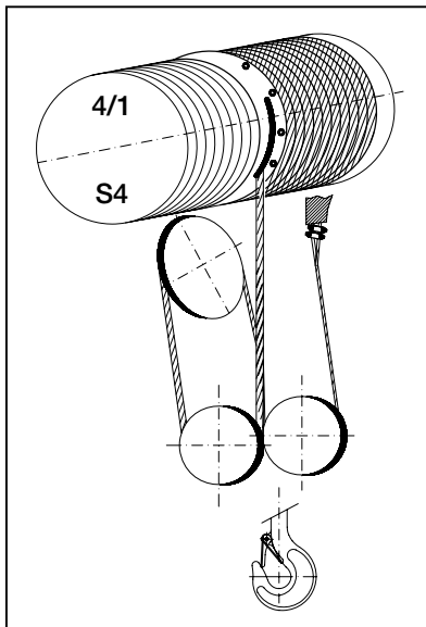
S4 - 4 TRAÇÕES DE CABO (4/1)
