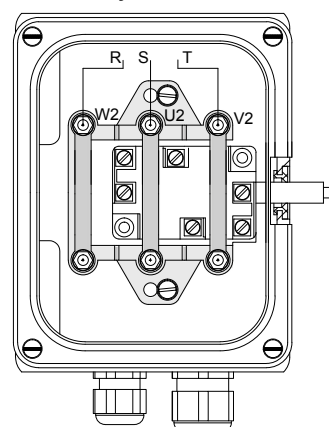
MOTOR COM DUPLA VELOCIDADE ALIMENTAÇÃO 220V 3PH
