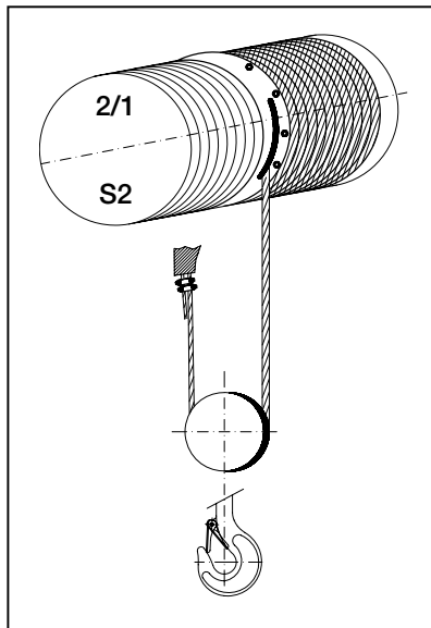
S2 - 2 TRAÇÕES DE CABO (2/1)
