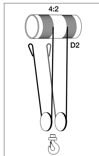
D2 - 4 WIRETALJER (4/2) MIDTERTRÆK
