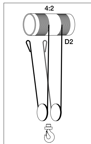
D2 - 4 TIRI DI FUNE (4/2) TIRO CENTRATO
