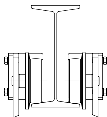
Binari ribassati - IPN, ecc. Underslung rails - IPN, etc.
